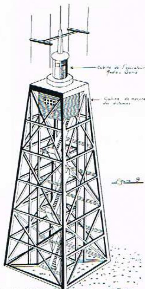
Pylône de récepteur Benito à moyenne portée
