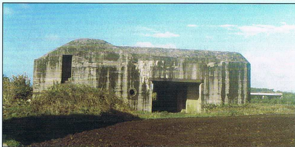
Ci-dessus : vue arrière d'une casemate H669 du Qu34 Keralland.
